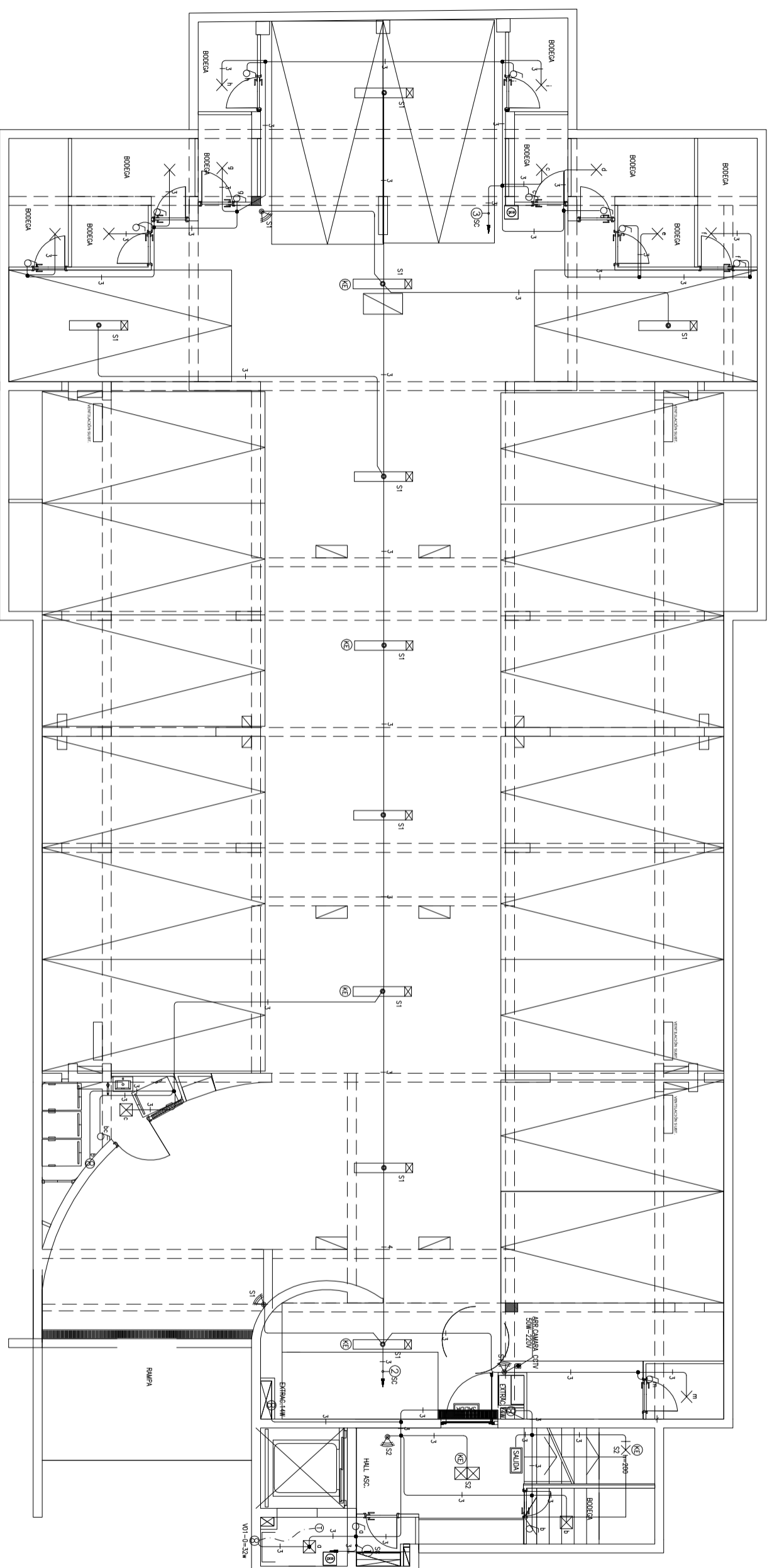
PLANTA PISO -1 ALUMBRADO ESC. 1 : 75
