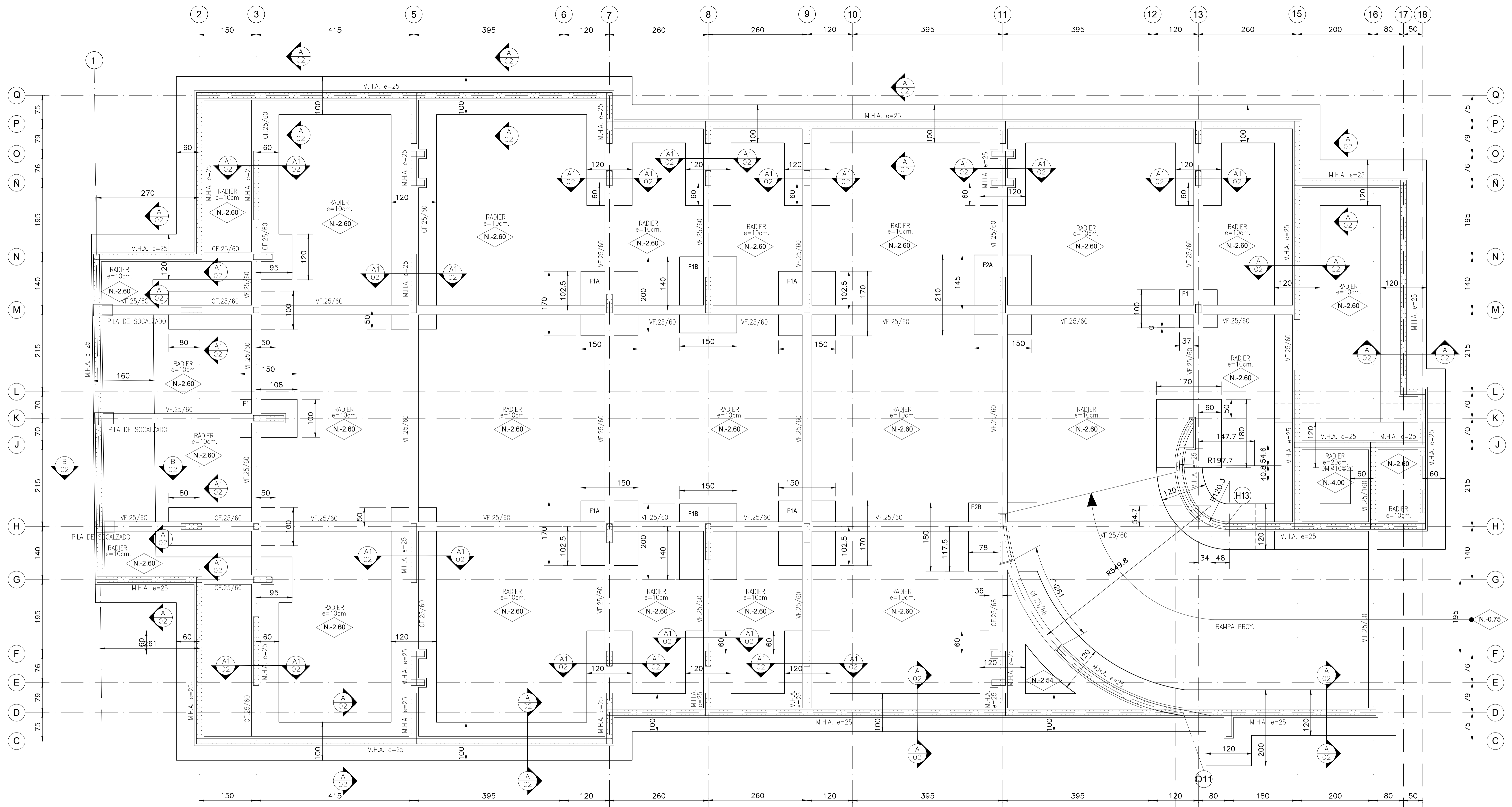
PLANTA FUNDACIONES S.F. -3.70m. ESC. 1:50 *VER PROYECTO ESPECIFICO PILAS DE SOCALZADO
