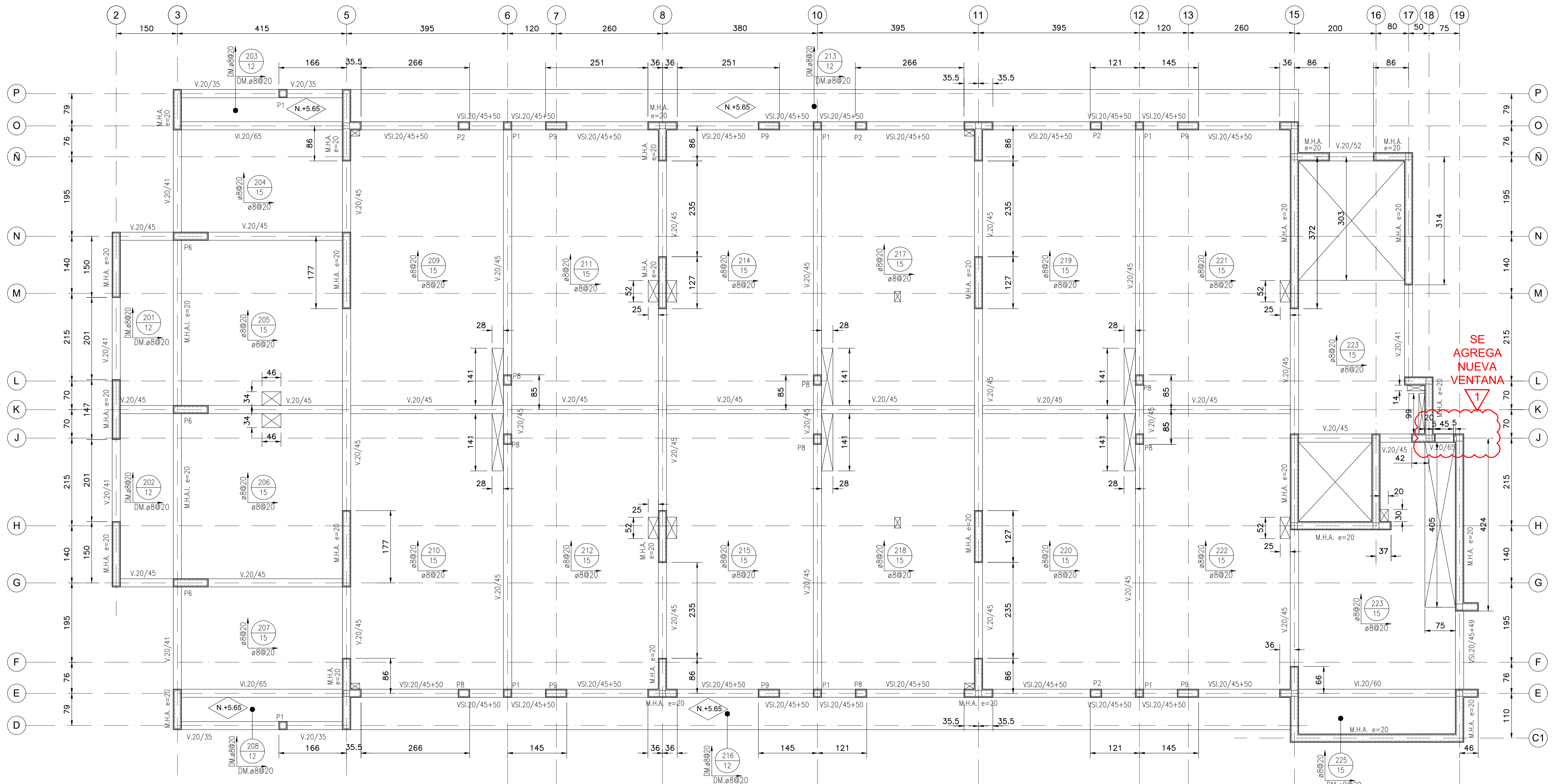
PLANTA ESTRUCTURA N.+5.15m. (S.I.C.) ESC. 1:50
