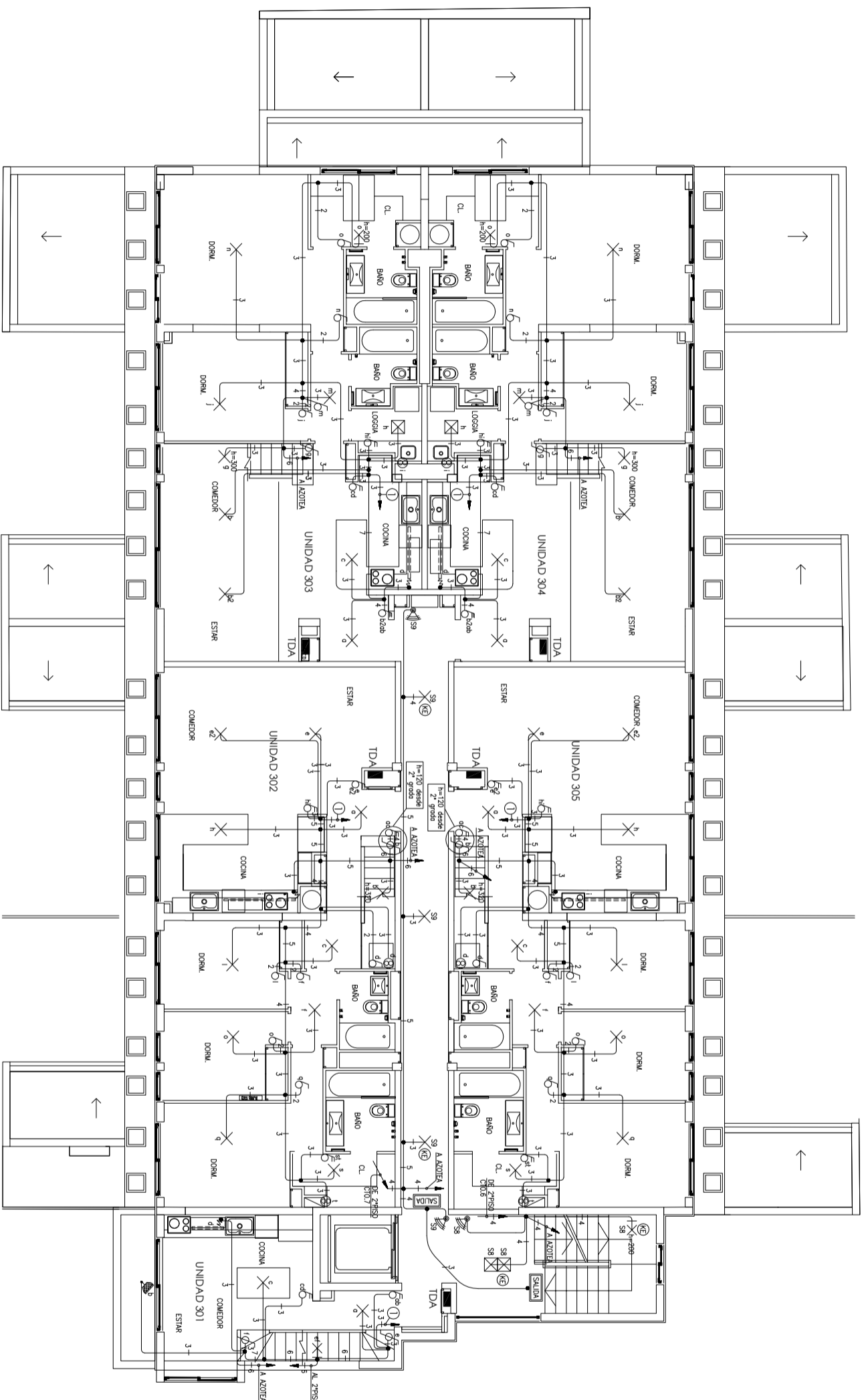
PLANTA PISO 3 ALUMBRADO ESC. 1 : 75
