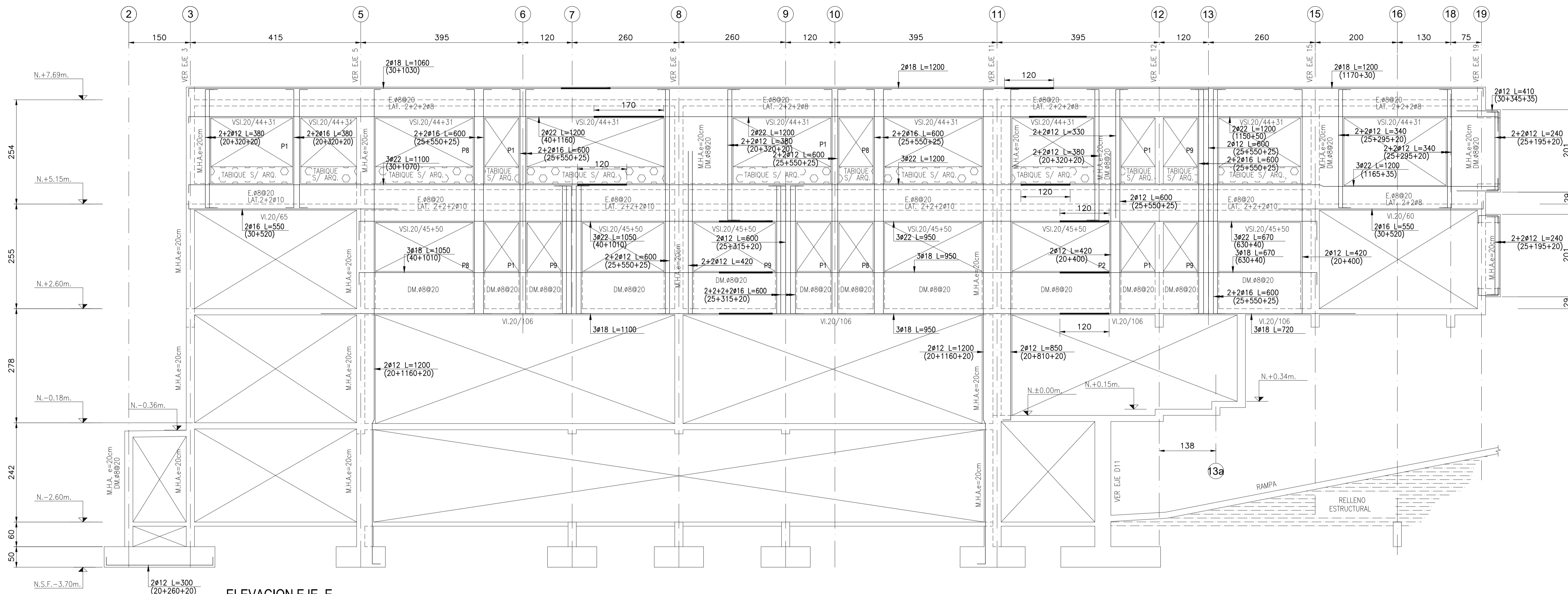
ELEVACION EJE E ESC. 1:50
