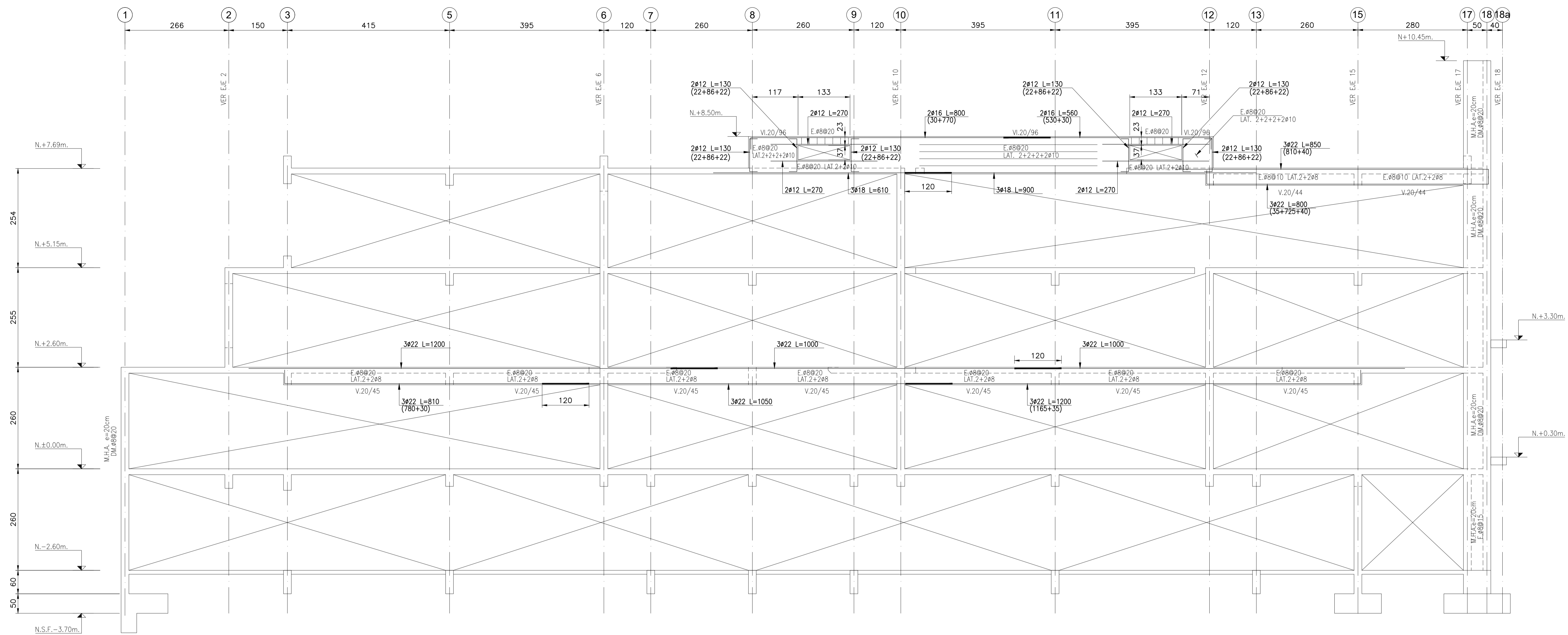
ELEVACION EJE L ESC. 1:50
