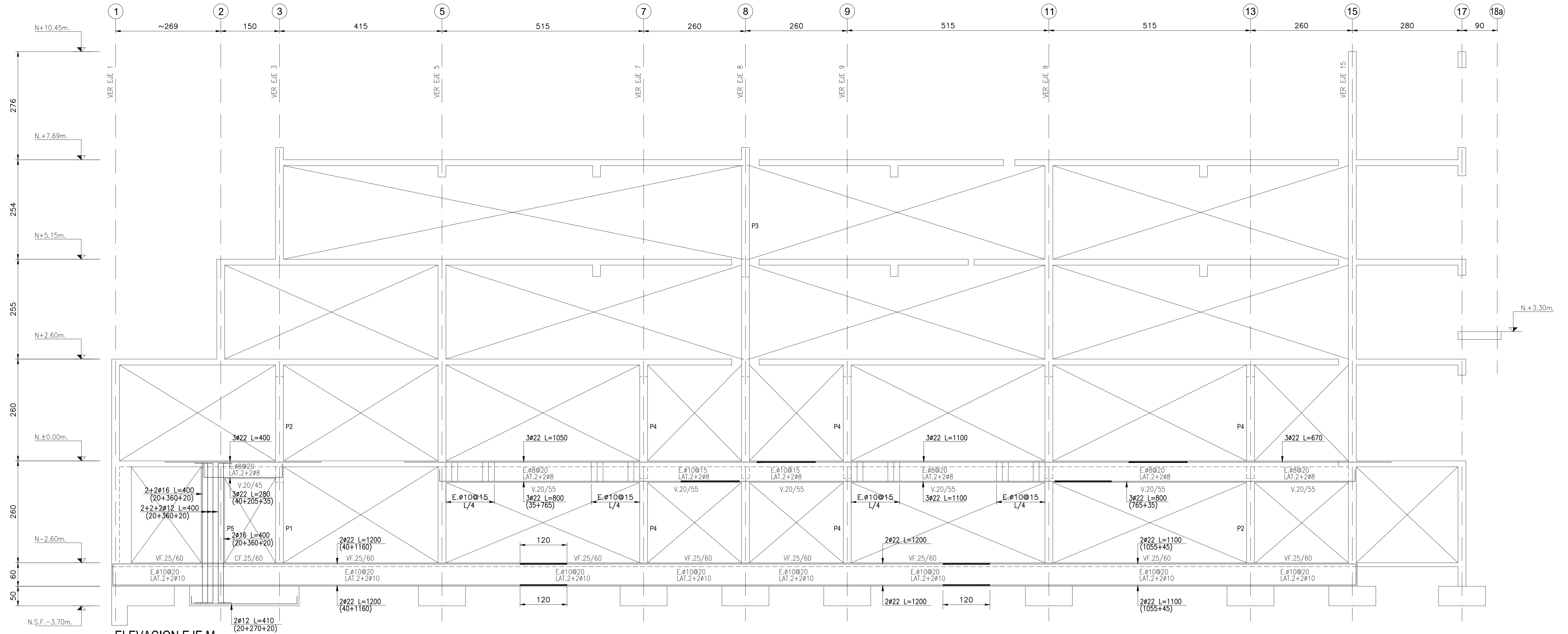
ELEVACION EJE M ESC. 1:50 *VER PROYECTO ESPECIFICO PILAS DE SOCALZADO
