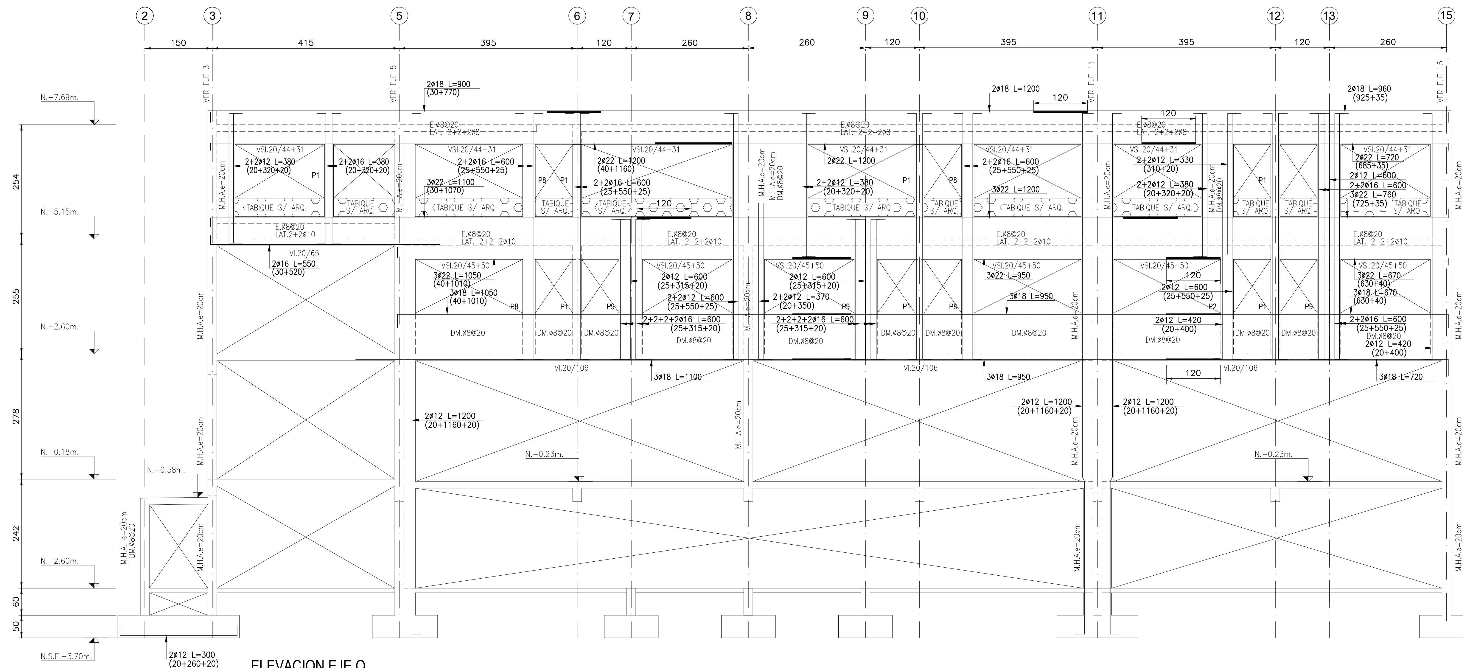
ELEVACION EJE O ESC. 1:50
