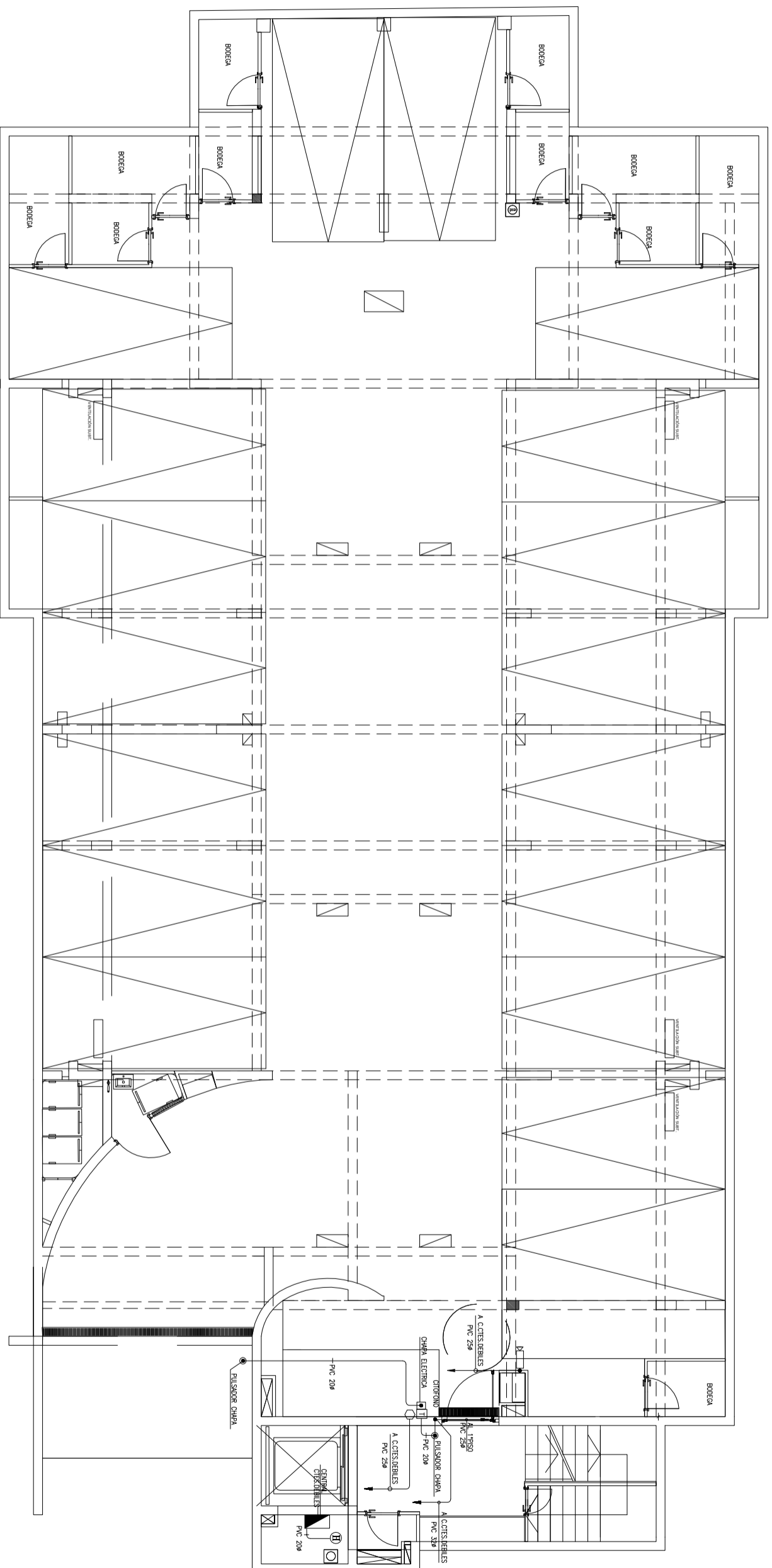
PLANTA PISO -1 C.TES. DEBILES ESC. 1 : 75
