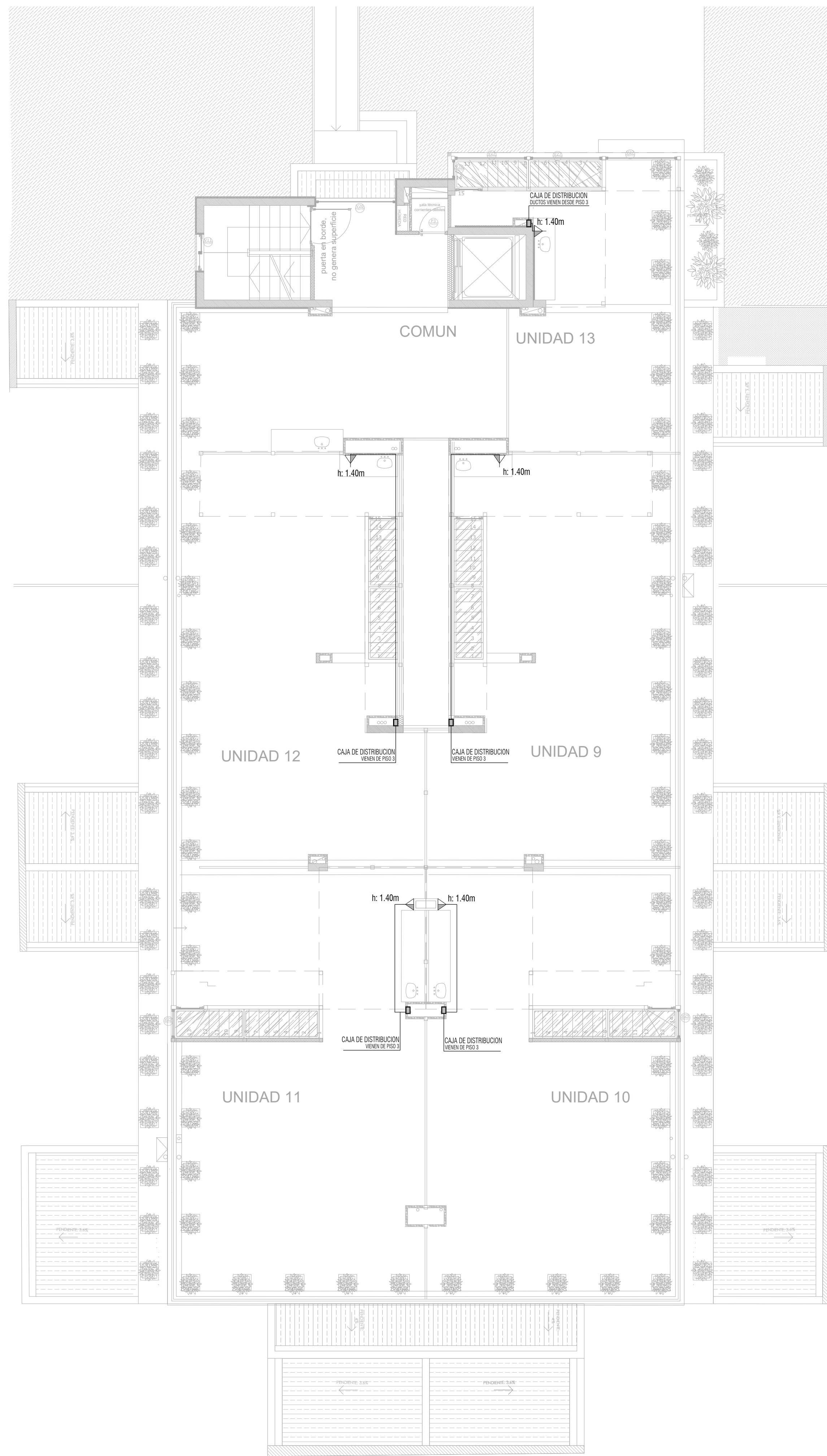
1 PLANTA TELECOMUNICACIONES PISO 4° 1:75
